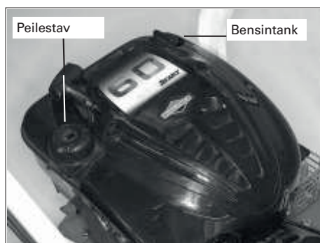
1) Bensin- og oljetank på B&S motor.
