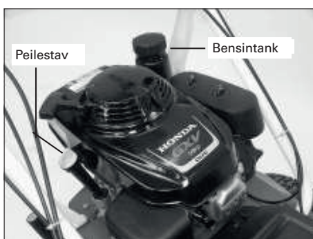
1) Bensin- og oljetank på Honda motor.
